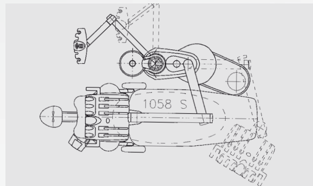
Van begin af aan perfect doordacht – horizontale projectie van de KaVo Primus S.
